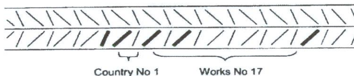
Obr.č.1: Identifikační číselný kód výrobce „Celsa „Huta Ostrowiec” Sp. z o.o.“
